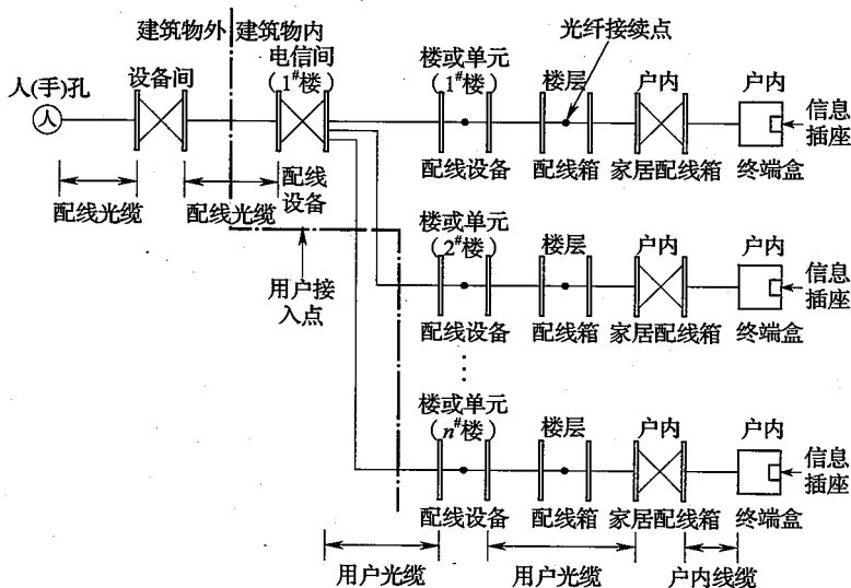
图 3 低层、多层、中高层住宅建筑用户接入点位置示意
